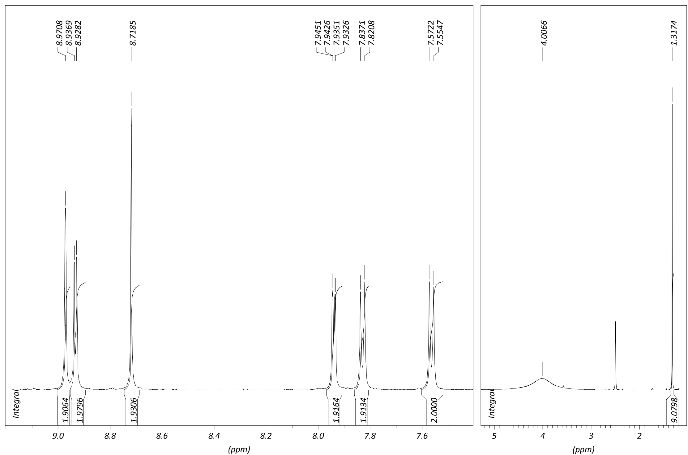
^1\text{H} -NMR-spectrum of 3
