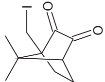
10-iodocamphorquinone_COSY.esp
